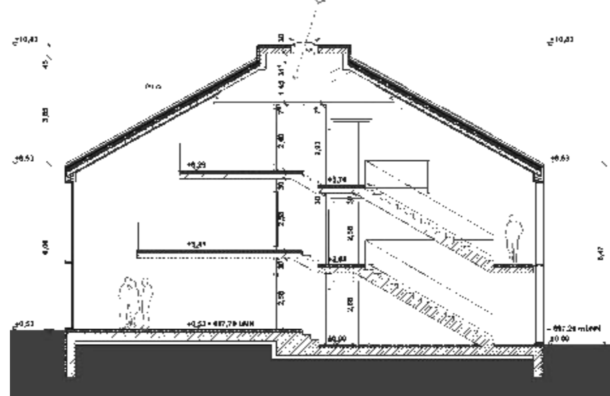
Schnitt B-B
