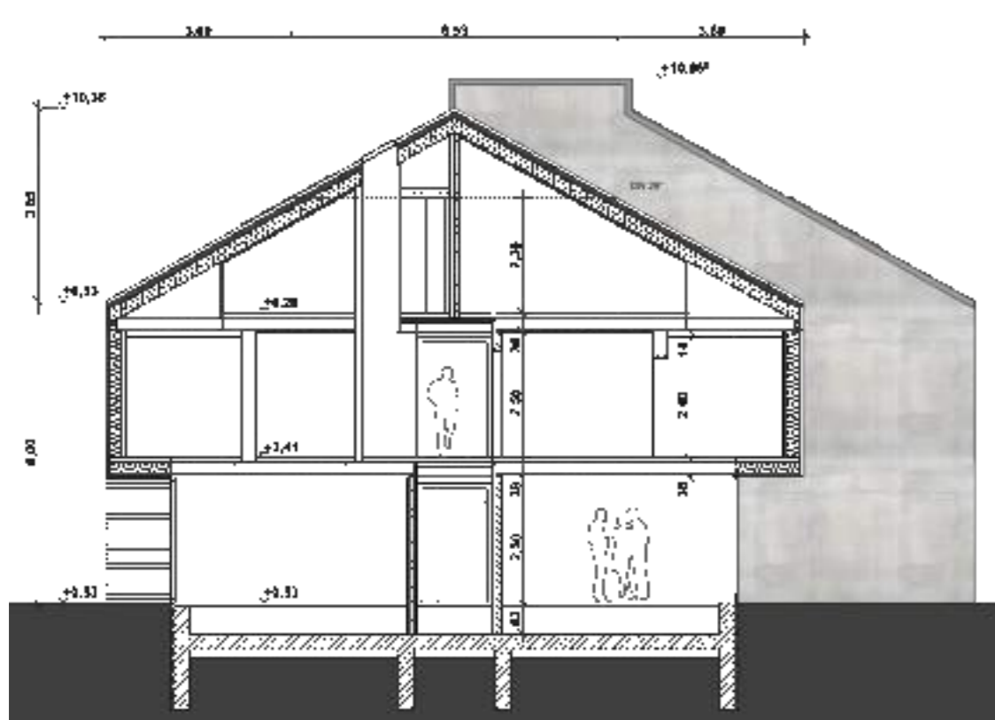
Schnitt A-A
