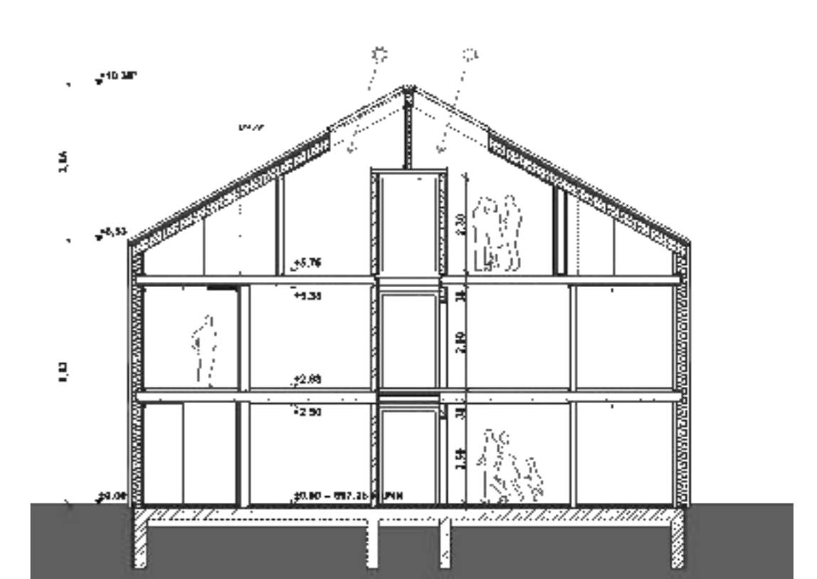
Schnitt C-C
