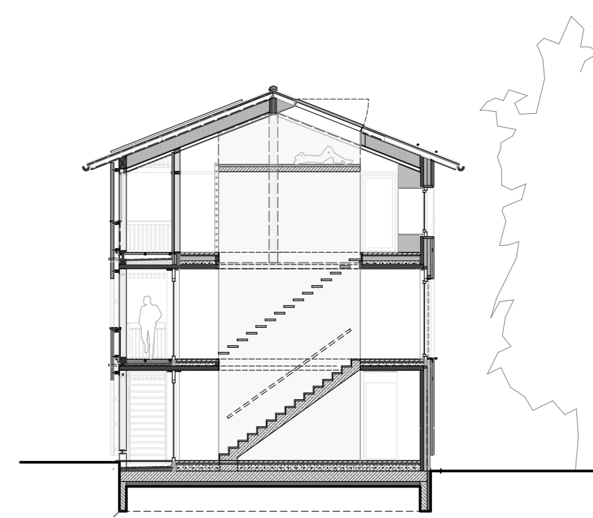
Schnitt und OG 5 m
